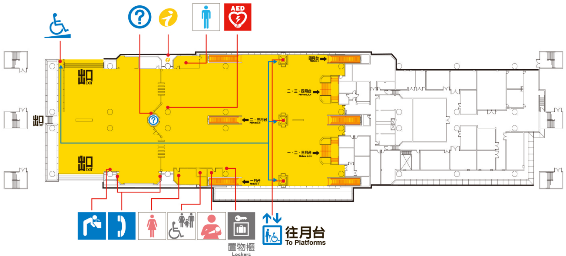
大廳層平面圖 Concourse Level
