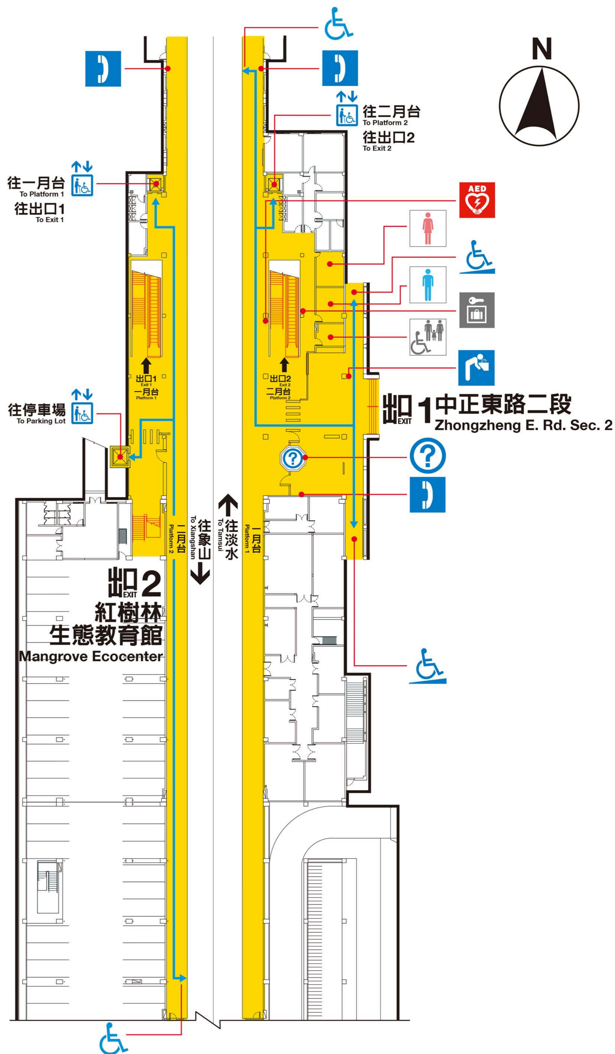
大廳/月台層平面圖 Concourse/Platform Level
