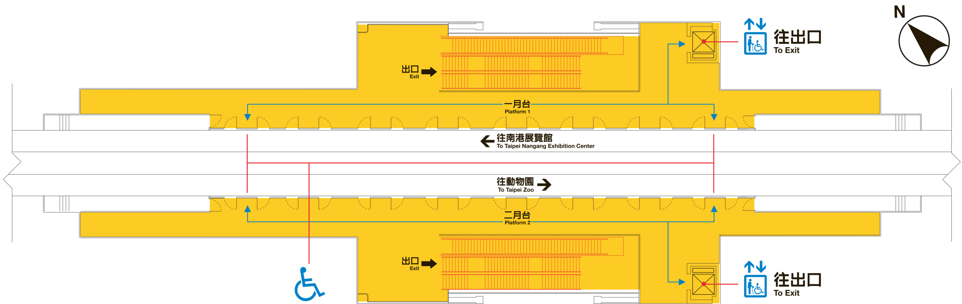
月台層平面圖 Platform Level
