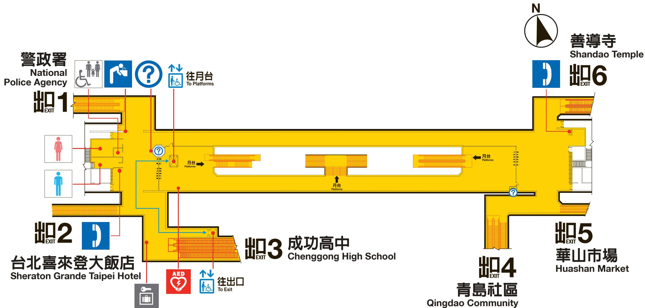
大廳層平面圖 Concourse Level
