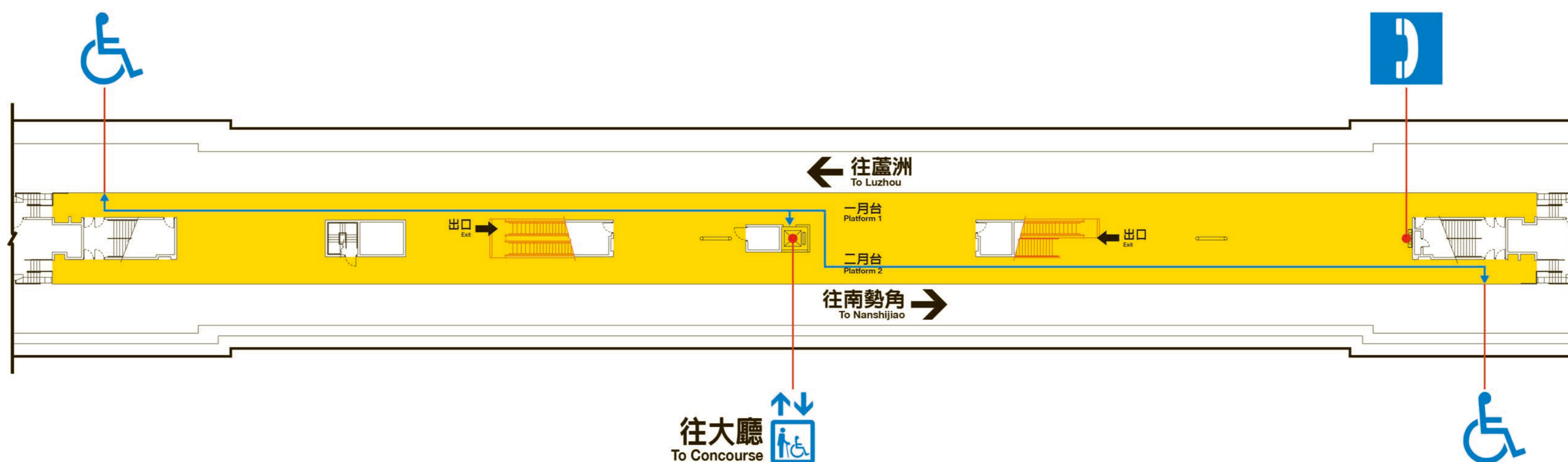
月台層平面圖 Platform Level
