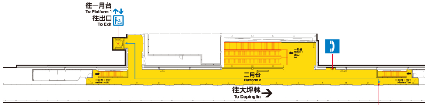
5F 上層月台平面圖 5F Upper Platform Level
