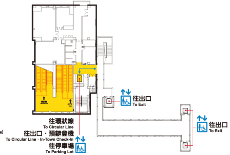
3F 連通道層平面圖 3F Passage Level
