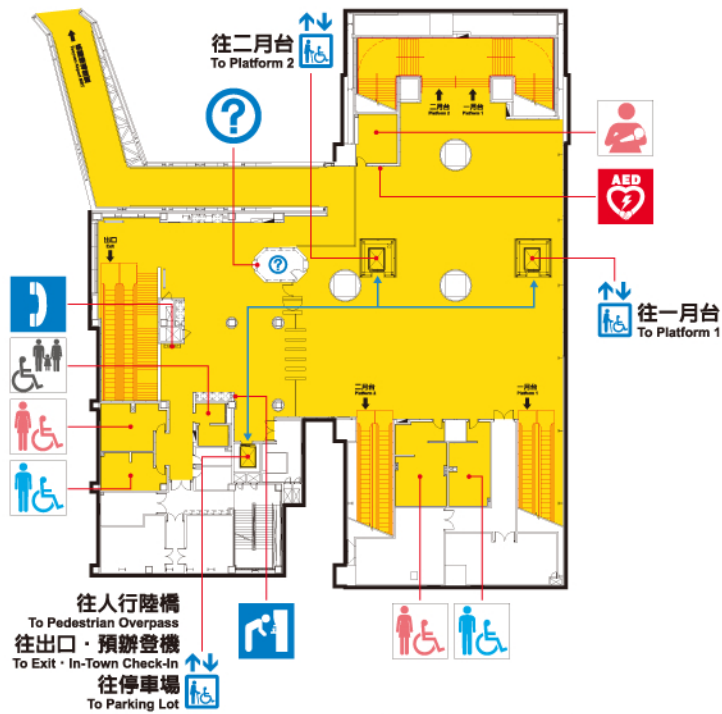
5F 大廳層平面圖 5F Concourse Level
