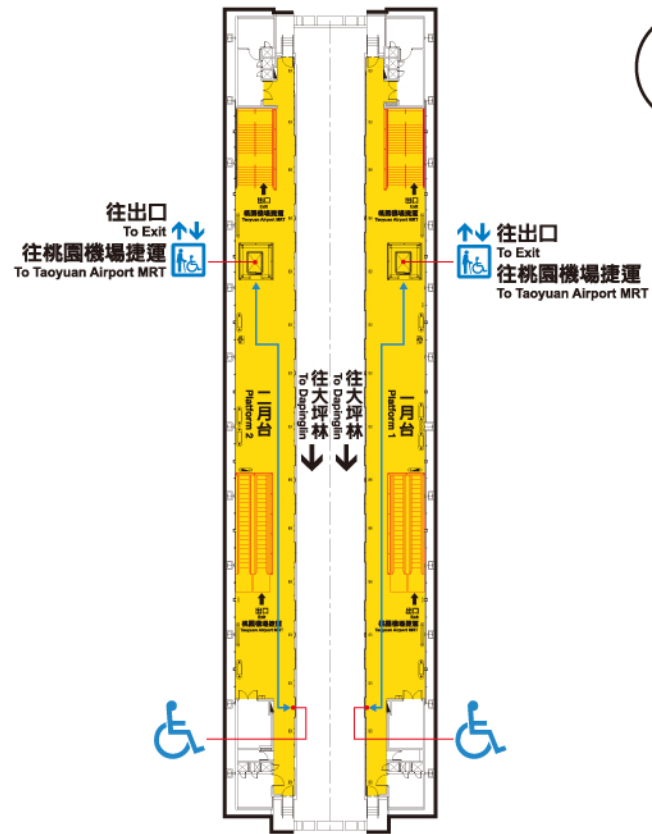
6F 月台層平面圖 6F Platform Level
